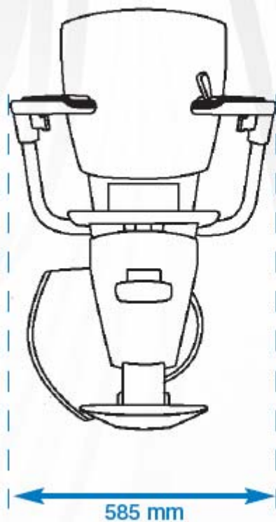
FRENTE – DESPLEGADA
