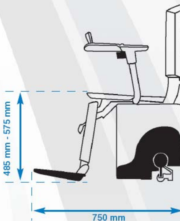
LADO – DESPLEGADA
